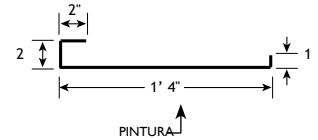
CABECERA DE PUERTA AL RAS FDH2 - Grosor 21"
