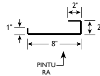
JAMBA DE PUERTA AL RAS FDJ2 - Grosor 13"
