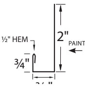
SOFFIT J-TRIM SJT - Girth 3.625"
