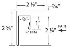
SOFFIT F&J SFJ - Girth 9.375"
